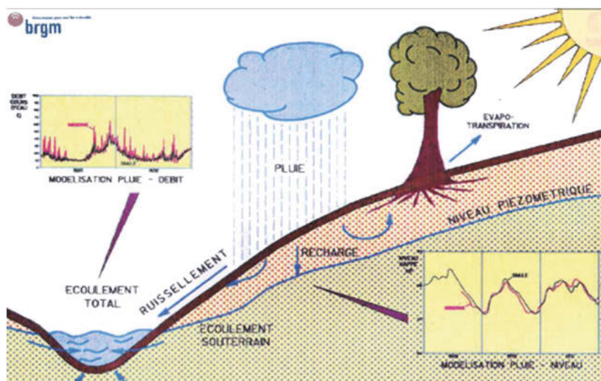
Figure 22 - Le fonctionnement d'un hydrosystème
