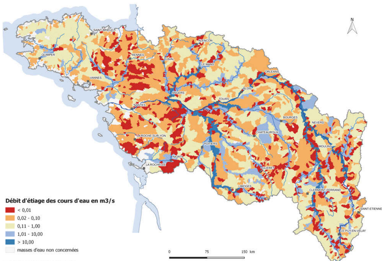
Carte 9 - Débits d'étiage observés des cours d'eau dans chacun des bassins versants de masse d'eau cours d'eau
