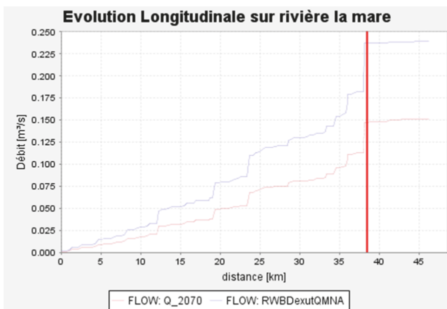
Graphique 37 - Débit potentiel de la rivière La Mare vers 2070
