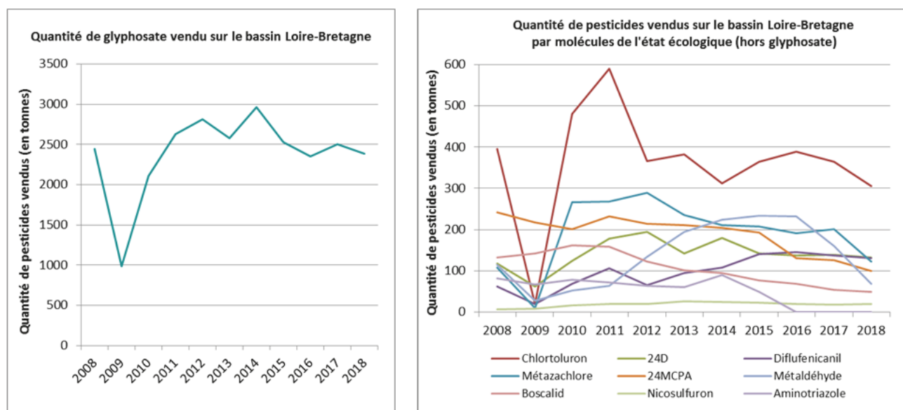
Graphiques 44 - Evolution de la quantité de pesticides vendue sur le bassin Loire-Bretagne par molécule de l'état écologique de 2008 à 2018 - Avec glyphosate (source : données de la BNV-d)
