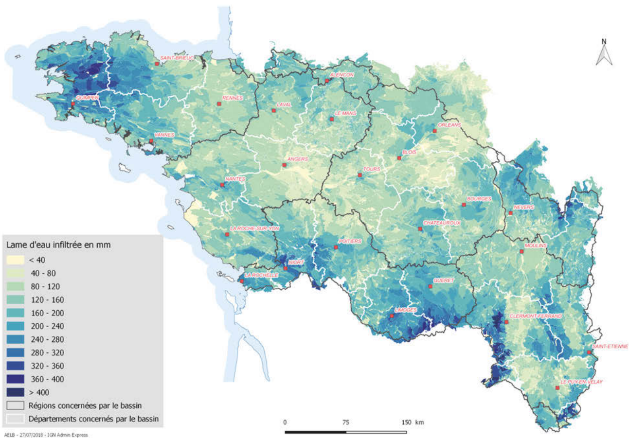
Carte 12 - Lames d'eau infiltrées (moyenne interannuelle en mm)
