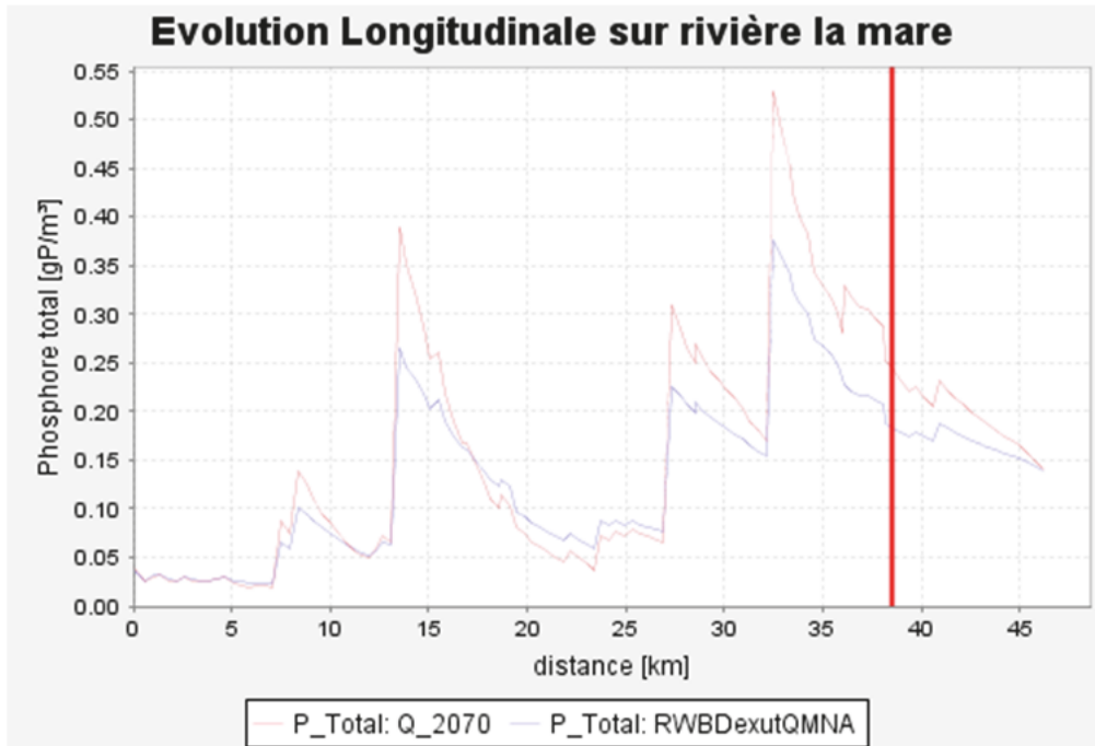
Graphique 38 - Concentration potentielle en phosphore total dans la rivière La Mare vers 2070
