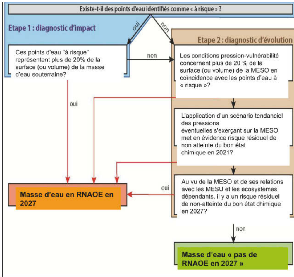
Figure 21 – Diagramme d'identification des masses d'eau souterraines à risque chimique
