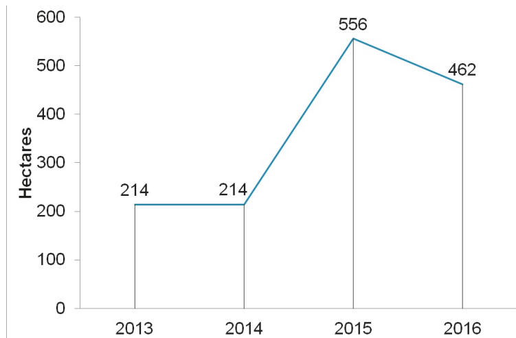
Graphique 6 - Évolution de la production d'algues (2013-2016)
