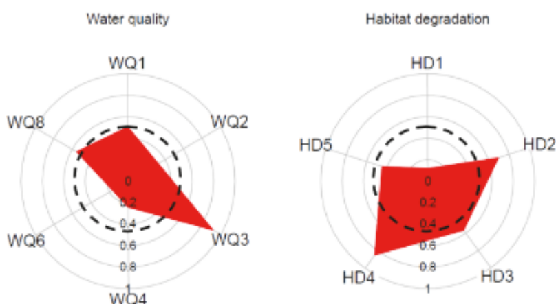
Graphique 53 - Exemple de cours d'eau impacté par les nitrates (WQ3), par une altération de sa ripisylve (HD2) et par un risque de colmatage (HD4)
