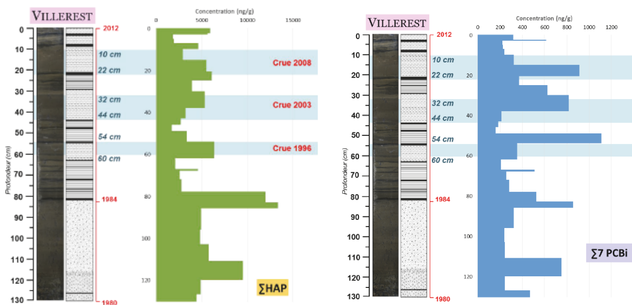
Figure 16 - Profil de distribution de la somme des HAP et de la somme des 7 PCB indicateurs selon la profondeur dans la retenue de Villerest
