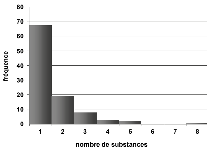
Graphique 19 - Distribution du nombre de substances non ubiquistes déclassantes par masse d'eau
